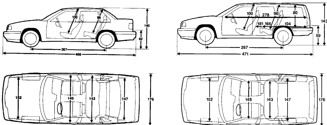
Abmessungen Volvo 850
